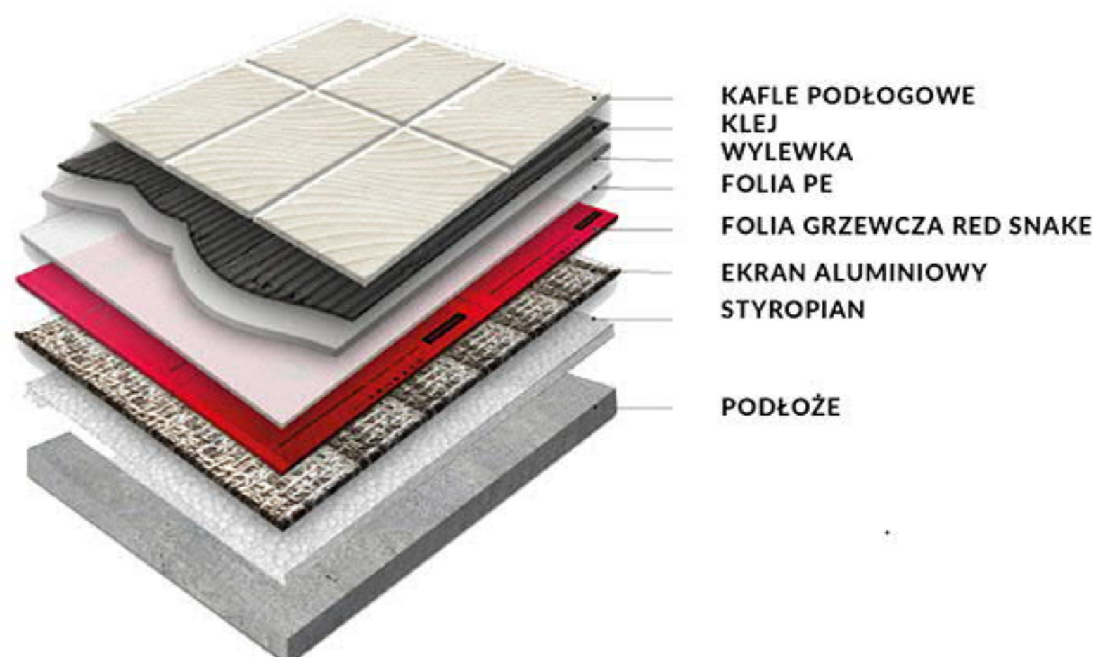
SCHEMAT UŁOŻENIA NA PODŁODZE Z PŁYTKAMI
