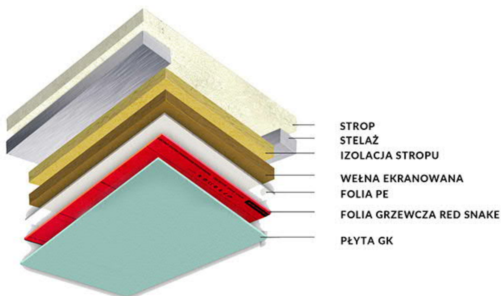
SCHEMAT UŁOŻENIA NA SUFICIE
